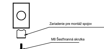
Demontáž Pohľad zhora
